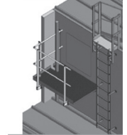
Plateforme sur toiture zinc Geh- plattform auf Zinkdach
