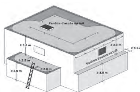
Sécurité en fonction des hauteurs et accès en toiture Sicherung entsprechend der Dachhöhe und -Zugang
